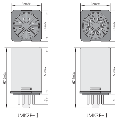
Dimensiones
